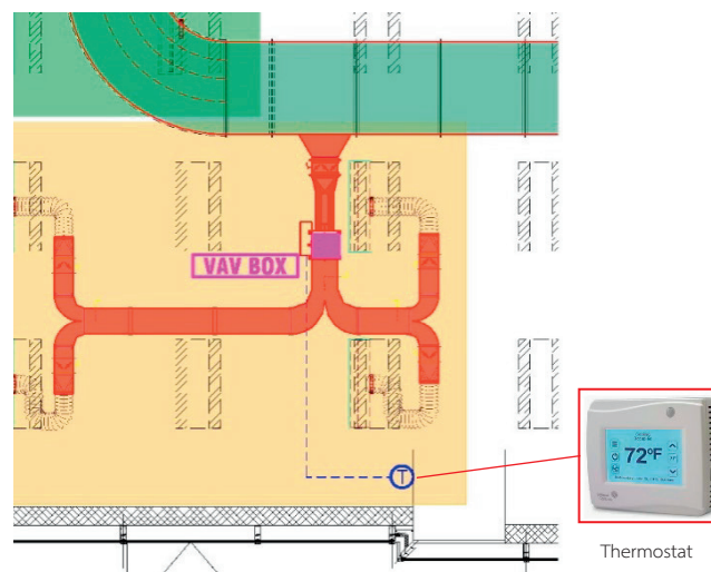
รูปที่ 50 การใช้อุปกรณ์ชุดควบคุมอุณหภูมิและปริมาณลม (thermostat) สำหรับ VAV box แต่ละชุด
