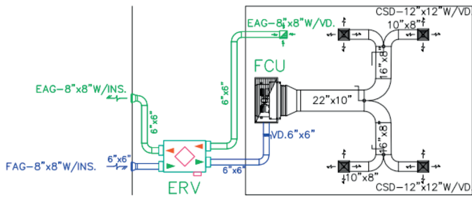
รูปที่ 67 ระบบการเติมอากาศกรณีที่ใช้ FCU แบบต่อท่อลม
