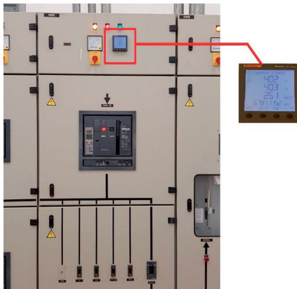
รูปที่ 72 ตัวอย่างการติดตั้งมาตรวัดไฟฟ้าหลักของอาคาร
