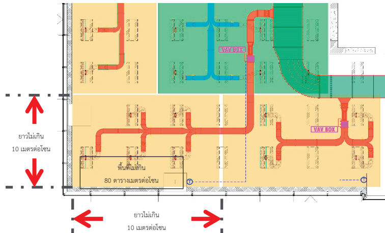
รูปที่ 49 การกำหนดโซนพื้นที่ใช้งานแต่ละโซนไม่เกิน 80 ตารางเมตร
