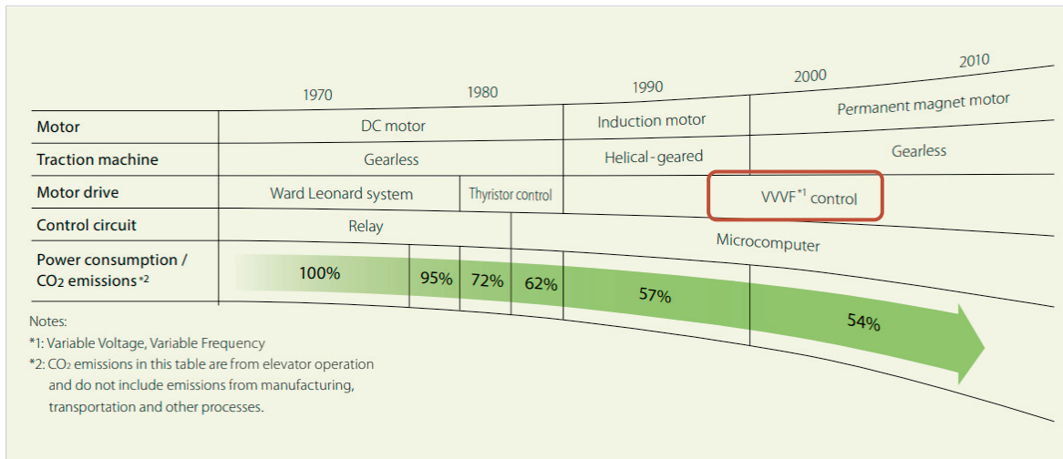
รูปที่ 69 ตัวอย่างการระบุคุณสมบัติการประหยัดพลังงานด้วยระบบควบคุมแบบ VVF
